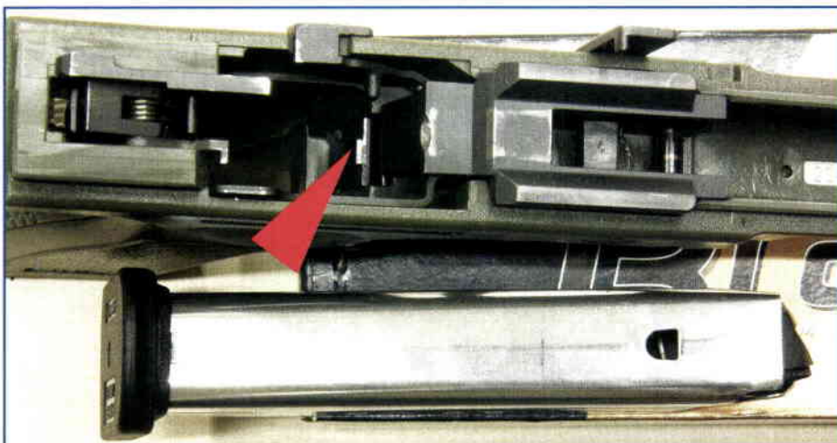
Záchyt zásobníku a drážka záchyty zásobníku v přední stěně zásobníku
